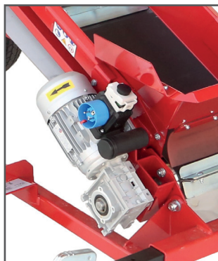
Elektrisches Förderband
